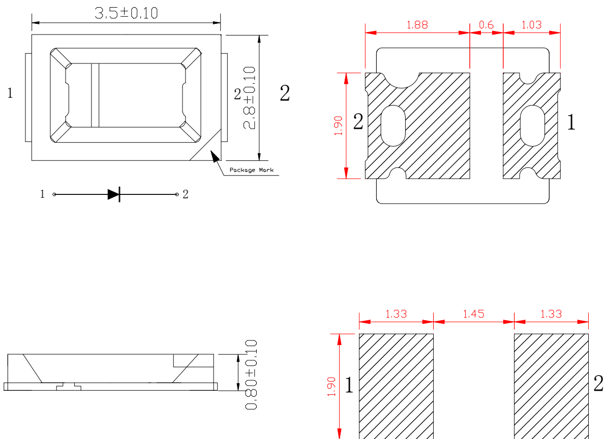
焊盘图
