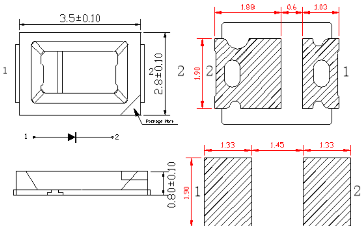
焊盘图
