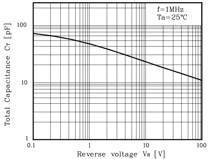
Fig. 4 C_J - V_R
