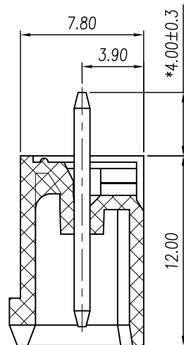
SECTION:A-A
