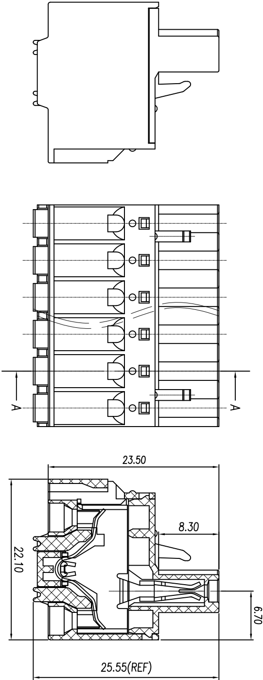
SECTION:A-A
