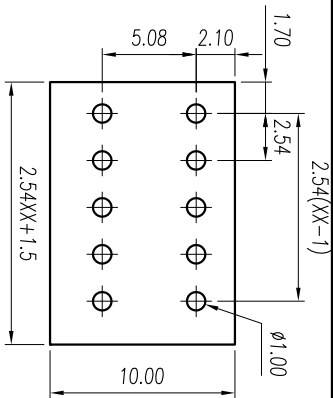
P.C.B. LAYOUT
