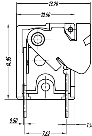
SECTION A-A P.C.B. LAYOUT
