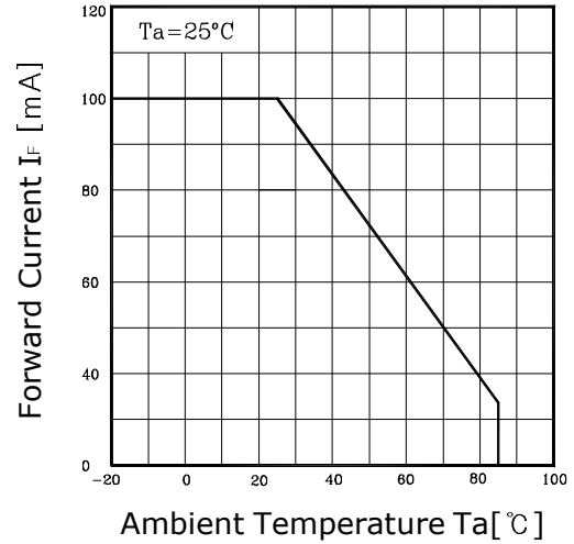
Fig.2 I_F - T_a
