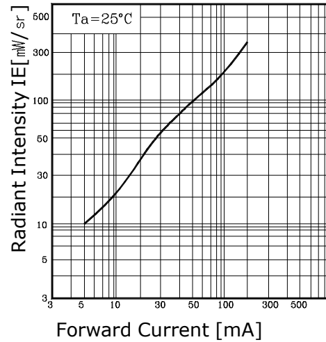
Fig.4 I_v - I_F
