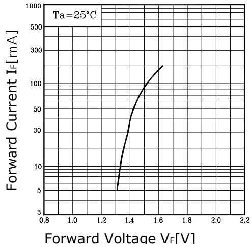
Fig.1 I_F - V_F
