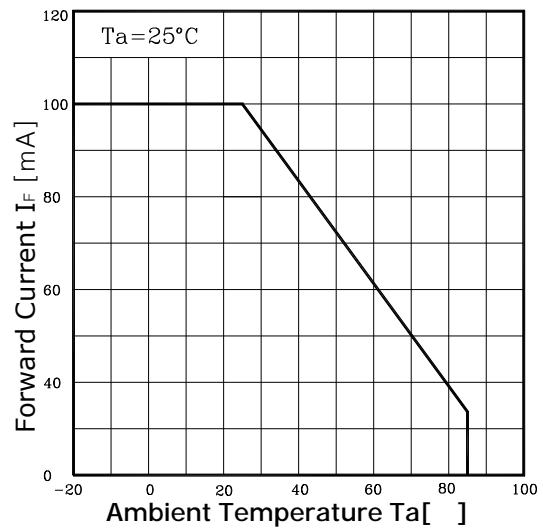
Fig.2 I_F - T_a
