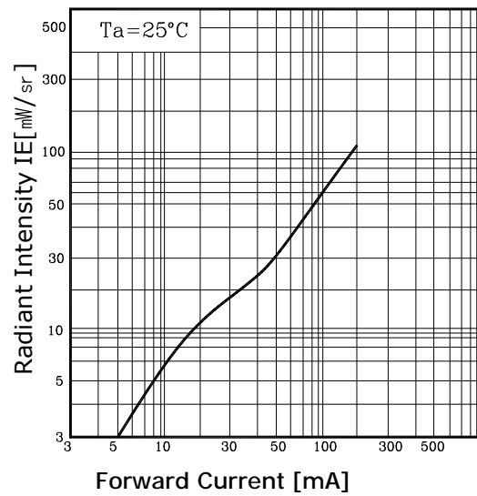
Fig.4 I_E - I_F
