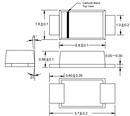
SOD - 123FL
