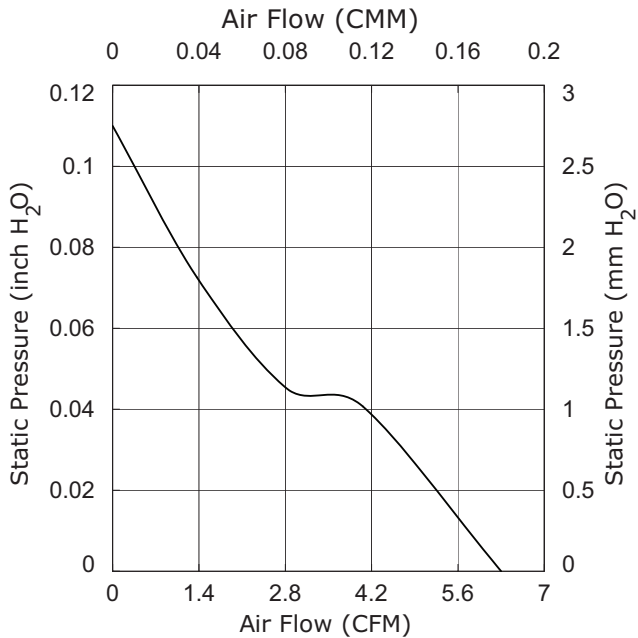
CFM-4020V-160-165
