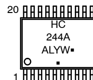
(TSSOP-20, TSSOP-20WB)
