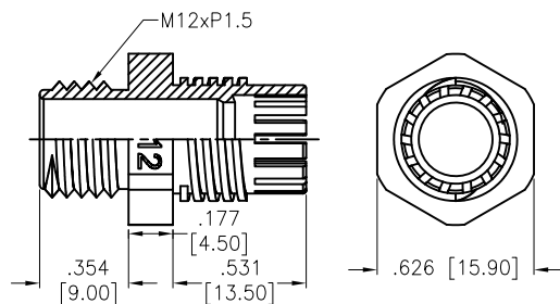
Ⓒ Body
