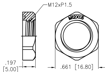
Ⓒ Body
