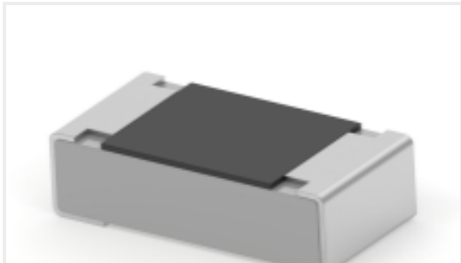
TE Part #1-2176340-9 CRGCQ 0603 1K0 5%
