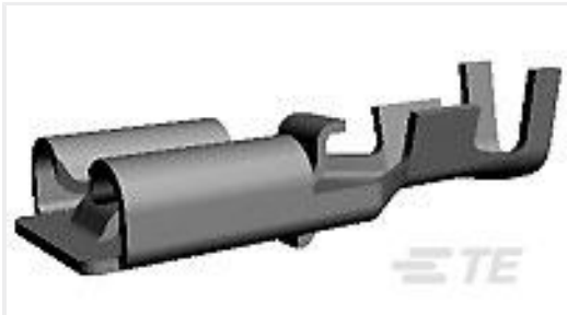
TE Part #626581-1 PL 250 REC 0.5-1.5 MM2 0.35X 26.54 BR
