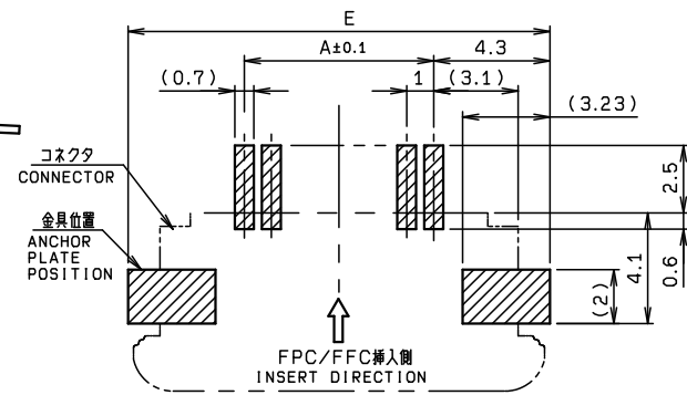
取付け基板寸法 (コネクタ搭載側) MOUNTING LAYOUT
