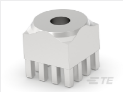
TE Part #225694-E POWELM BUCHSE ZWEIM M4 6 2,54 * EP 7 CUS
