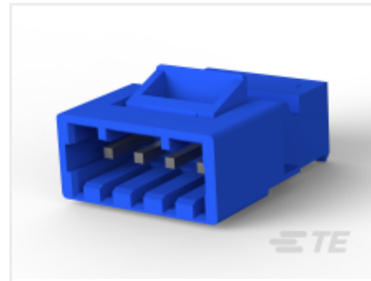
TE Part # 3-641439-4 04P MTA156 PST CON ASSY LF
