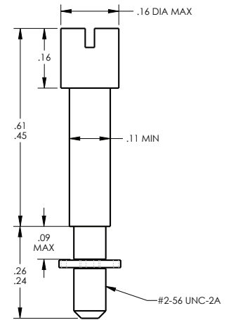
#2/56 DCJS9-51SLP
