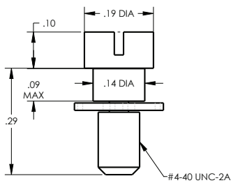
#4/40 DCJS100SLP
