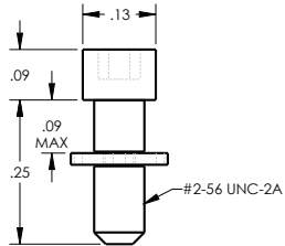
#2/56 DCJS9-51HLP
