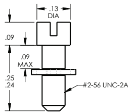
#2/56 DCJS9-51SLP
