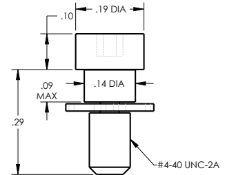
#4/40 DCJS100HLP
