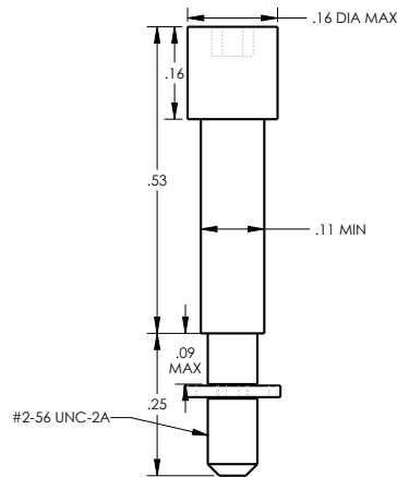
#2/56 DCJS9-51H
