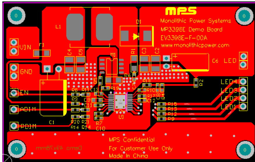
Figure 1—Top Layer
