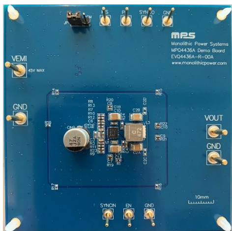
(LxWxH) 9cmx9cmx1.3cm
