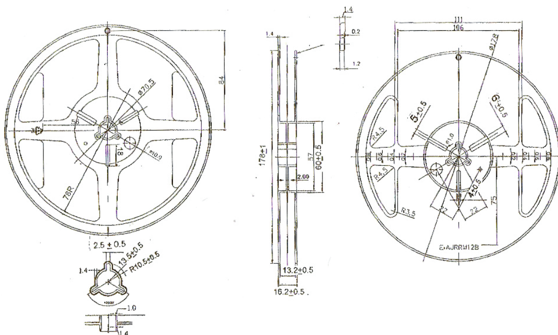
Fig. 12 - Reel Dimensions
