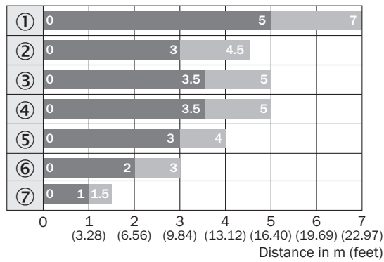
스위칭 거리 다이어그램 WL12-3
