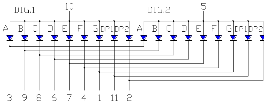
OPS-D2814 (Common Anode)
