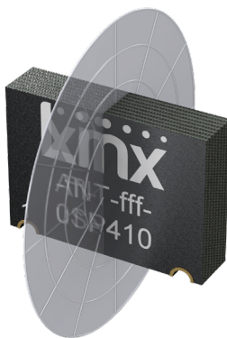
YZ-Plane Gain
