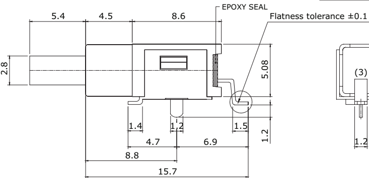
5.4 MM ACTUATOR
