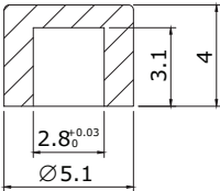
ACTUATOR CAP
