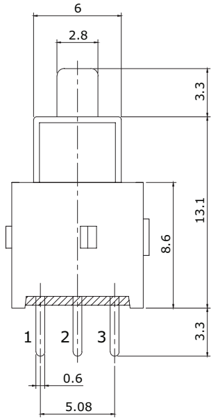
3.3 MM ACTUATOR
