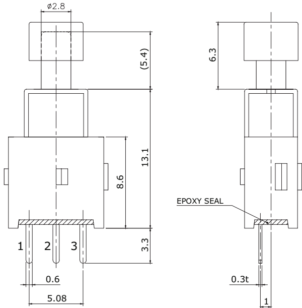
5.4 MM ACTUATOR
