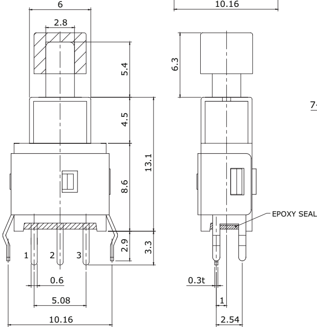
5.4 MM ACTUATOR
