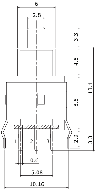
3.3 MM ACTUATOR
