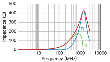
MMZ0603D800CT000
