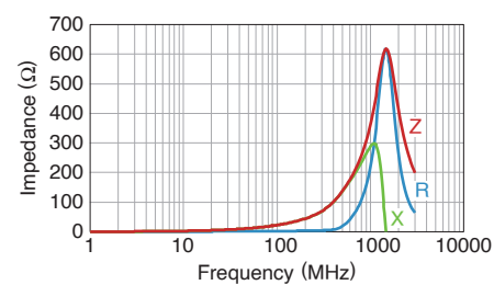
MMZ0603F220CT000
