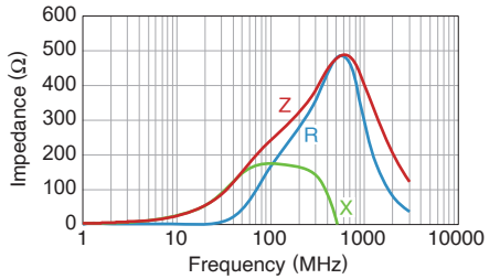
MMZ0603D330CT000
