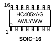
SOIC-16
