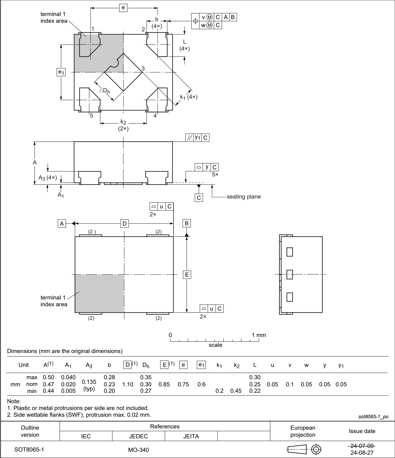
Fig. 27. Package outline SOT8065-1 (XSON5)
