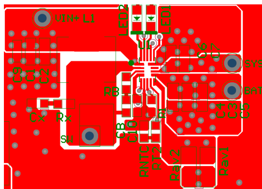
Top Layer
