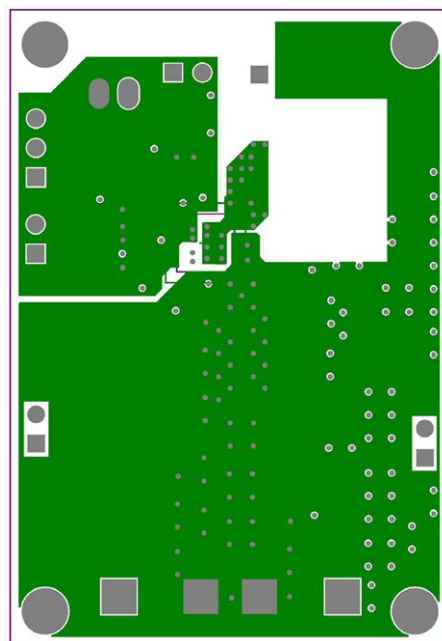
Fig. 44 - Inner Layer 2
