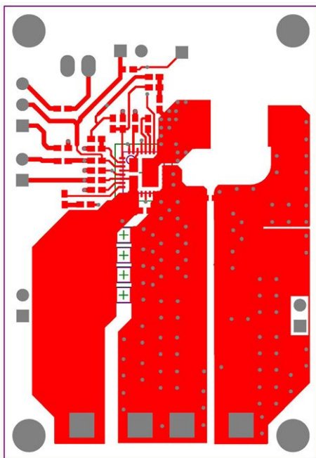
Fig. 42 - Top Layer
