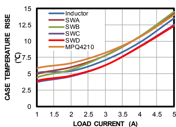
Thermal Rise
