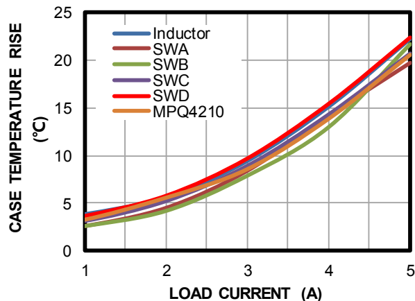
Thermal Rise
