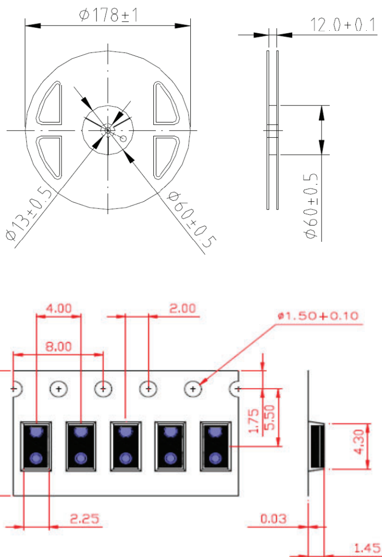
Fig. 16 - Reel Dimensions
