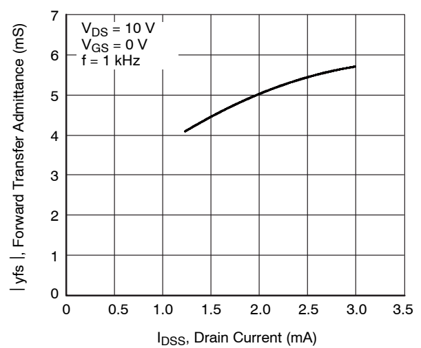
Figure 6. |y_{fs}| - I_{DSS}
