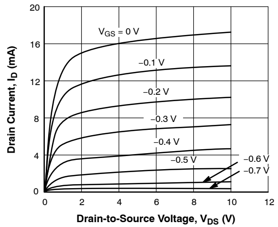
Figure 2. I_D - V_{DS}
