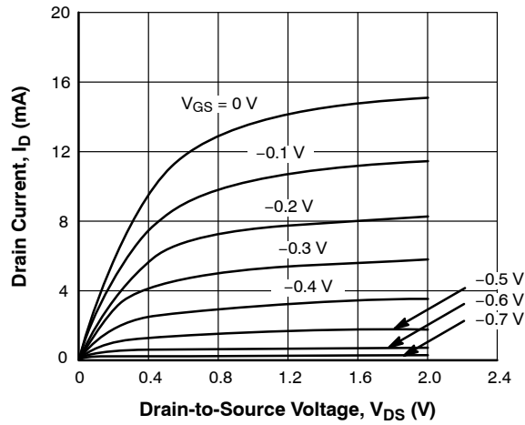
Figure 1. I_D - V_{DS}
