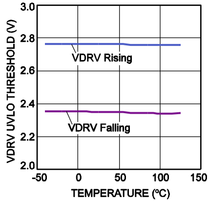
VDRV UVLO
