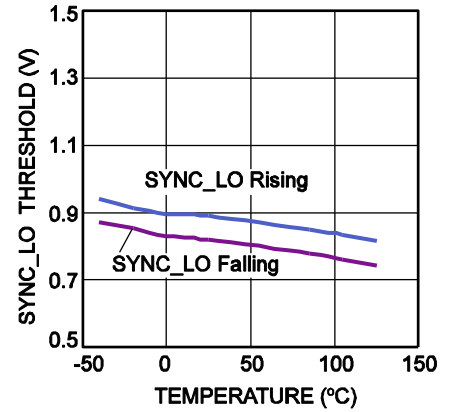
Sync_Lo
