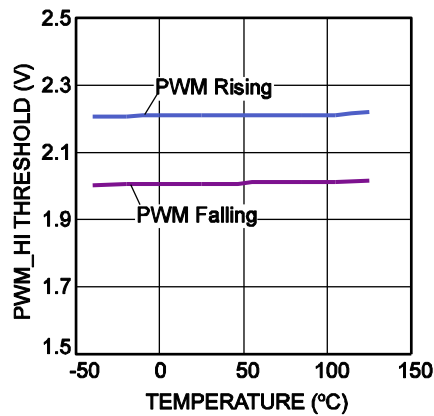
PWM Hi
