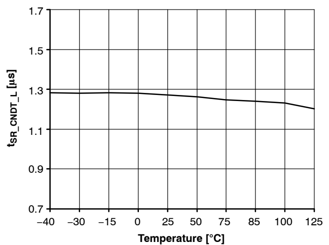
Figure 12. tSR_CNDT_L
